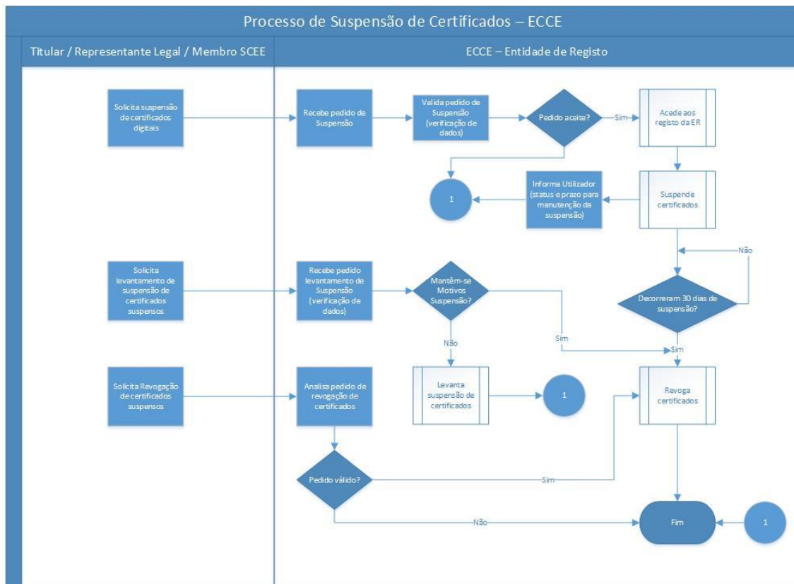
Figura 3 – Processo de Pedido de Suspensão de Certificados.
